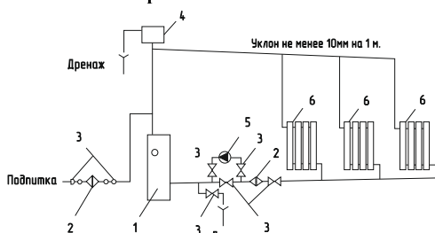
Схема открытой системы отопления
