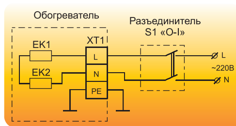
Схема электрическая принципиальная инфракрасного обогревателя IC-20
