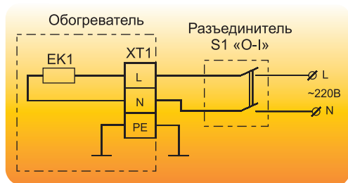
Схема электрическая принципиальная инфракрасного обогревателя IC-08, IC-10
