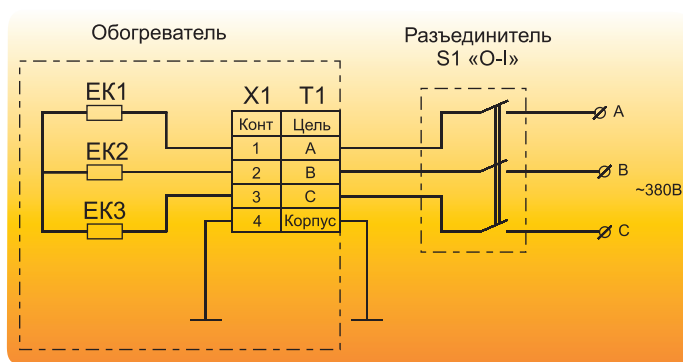
Схема электрическая принципиальная инфракрасного обогревателя IC-30, IC-40
