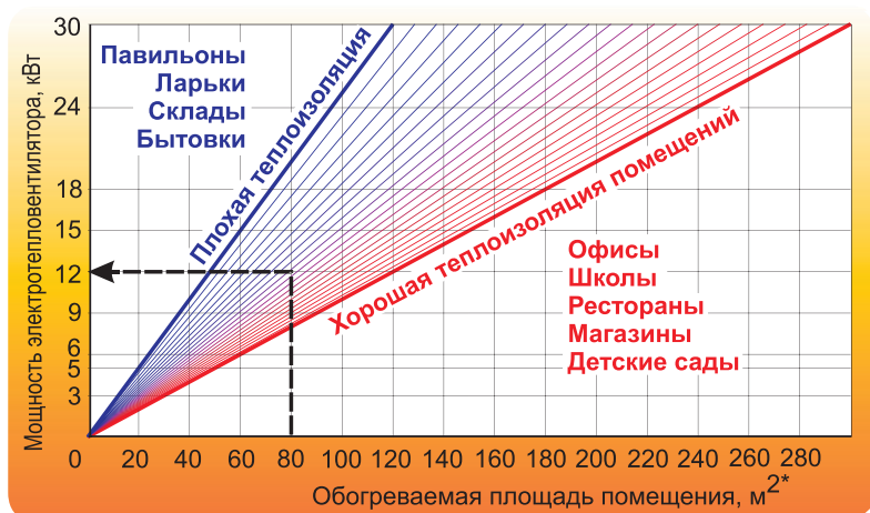
График 2. Определение необходимой мощности тепловентилятора серии T
