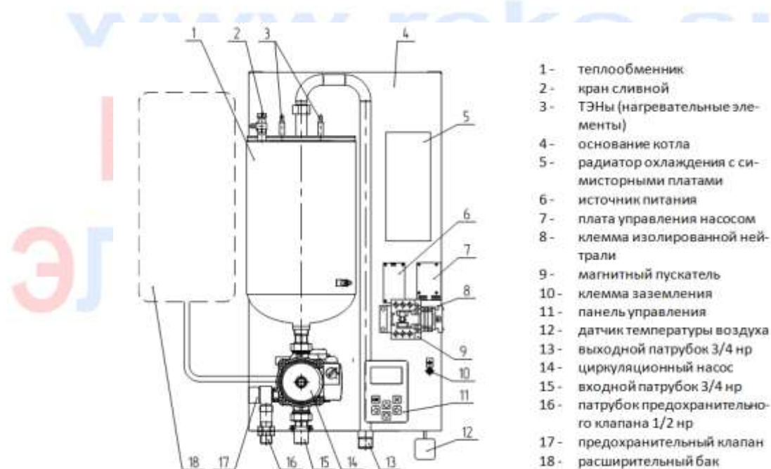
Рисунок 1. Устройство отопителя РЭКО серии П
