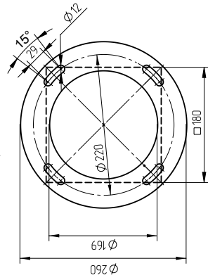
Фланец присоединительный
