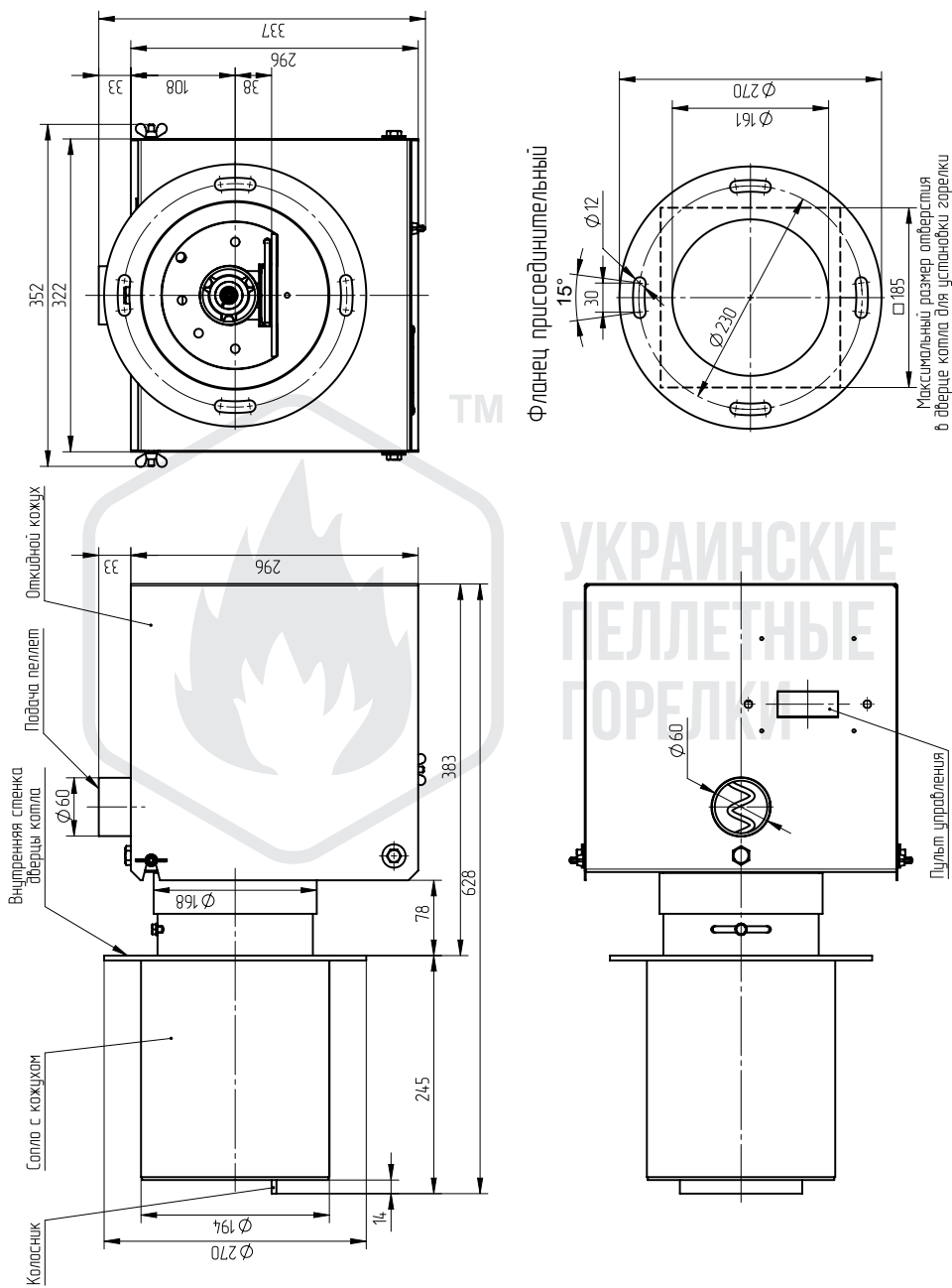
Рис.4 Габаритные размеры горелки LIBEATOR RCE-50(м)
